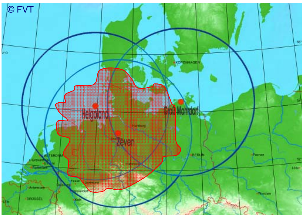
Bild 2: Berechnete Ausbreitung unter Berücksichtigung der Bodenleitfähigkeiten
