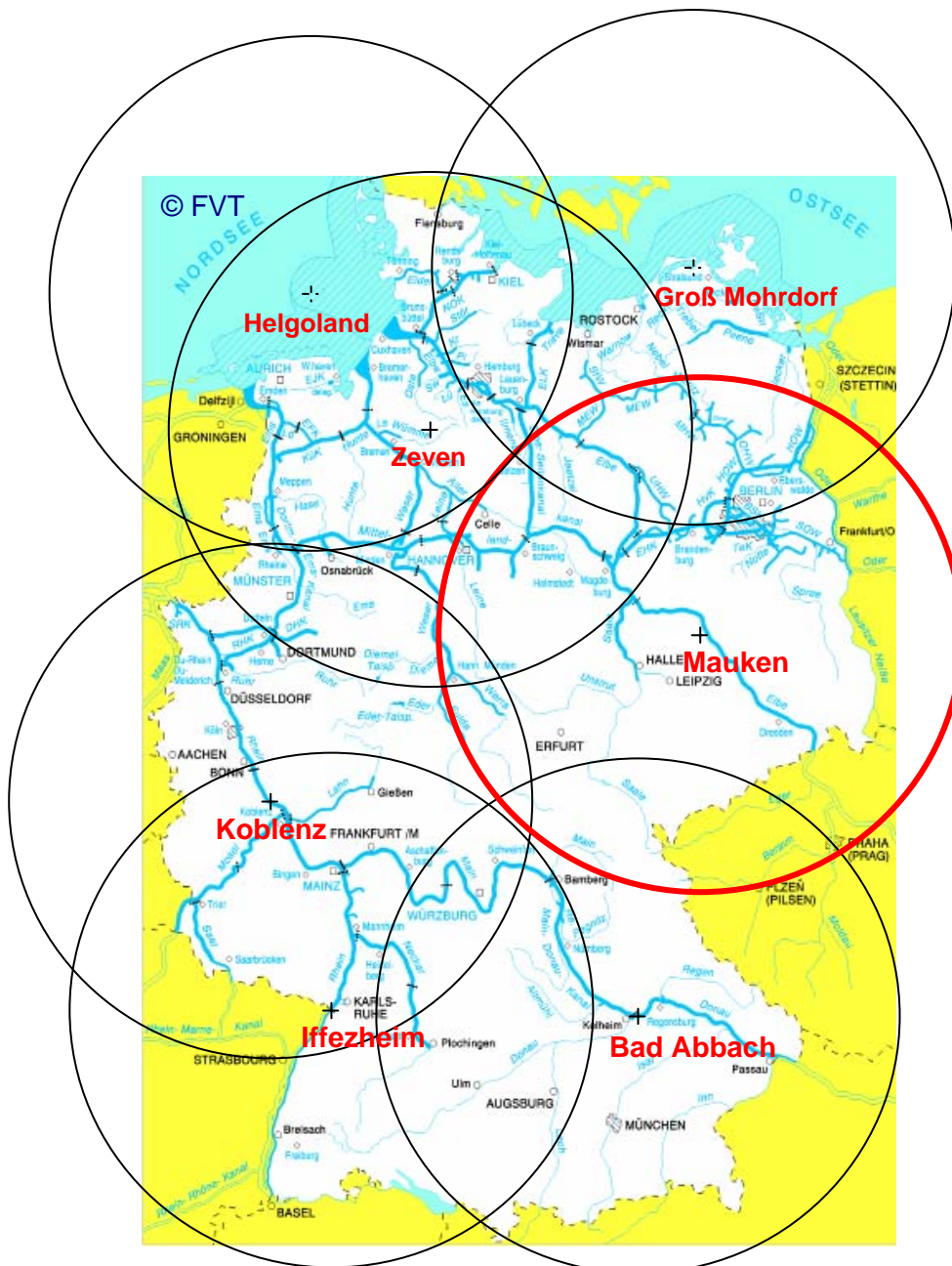
Bild 1: Einfache Reichweitendarstellung der deutschen DGPS-Referenzstationen in der Kreisform (In Rot DGPS Mauken)
