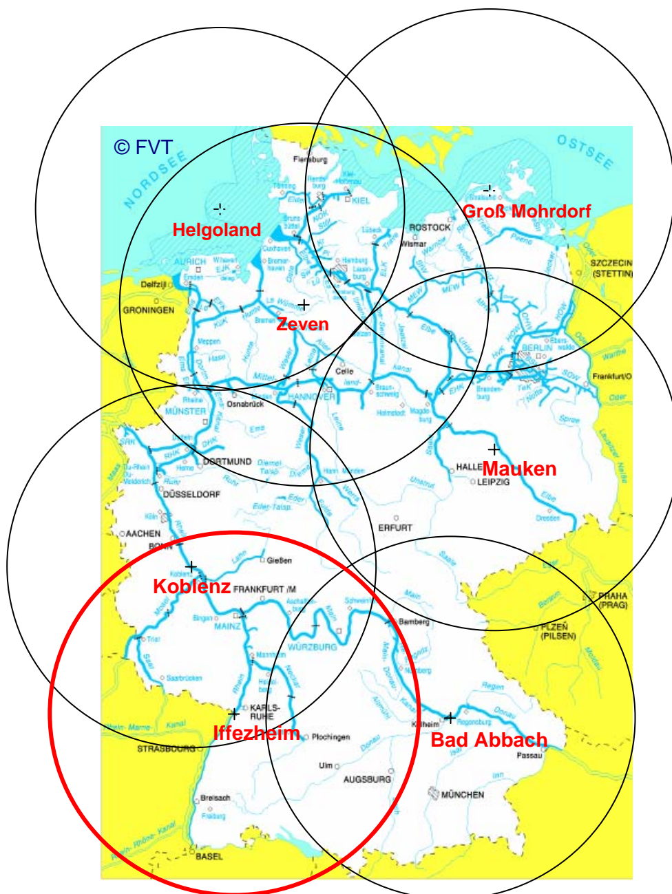
Bild 1: Einfache Reichweitendarstellung der deutschen DGPS-Referenzstationen in der Kreisform (In Rot DGPS Iffezheim)
