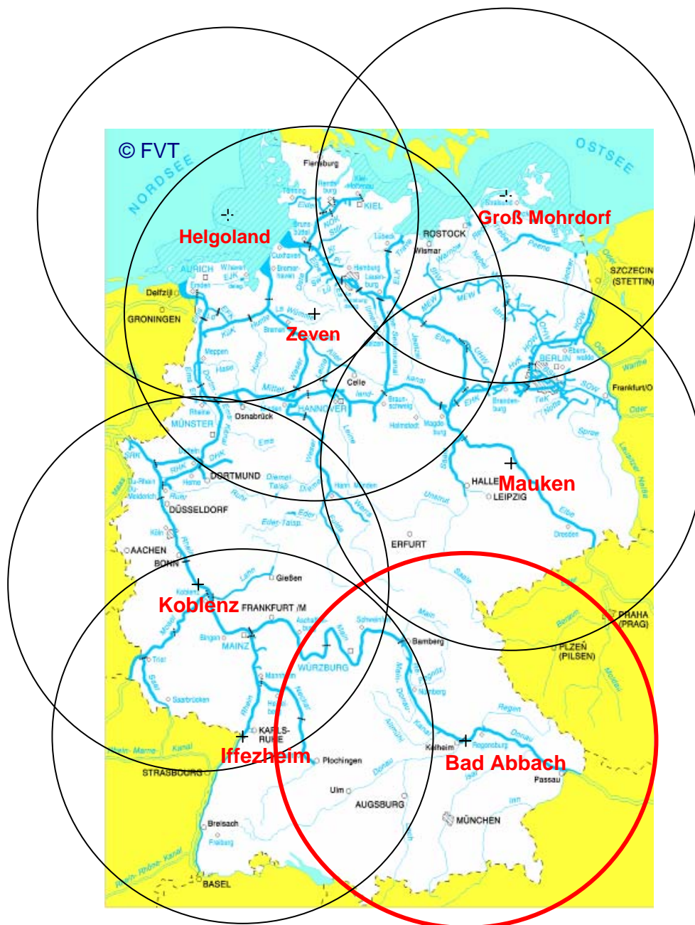
Bild 1: Einfache Reichweitendarstellung der deutschen DGPS-Referenzstationen in der Kreisform (In Rot DGPS Bad Abbach)
