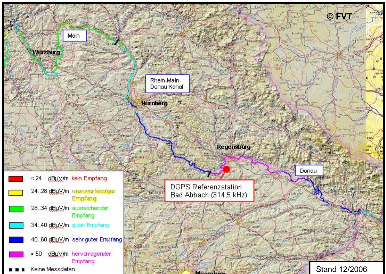
Bild 1: Empfangsfeldstärkewerte der DGPS Referenzstation Bad Abbach
